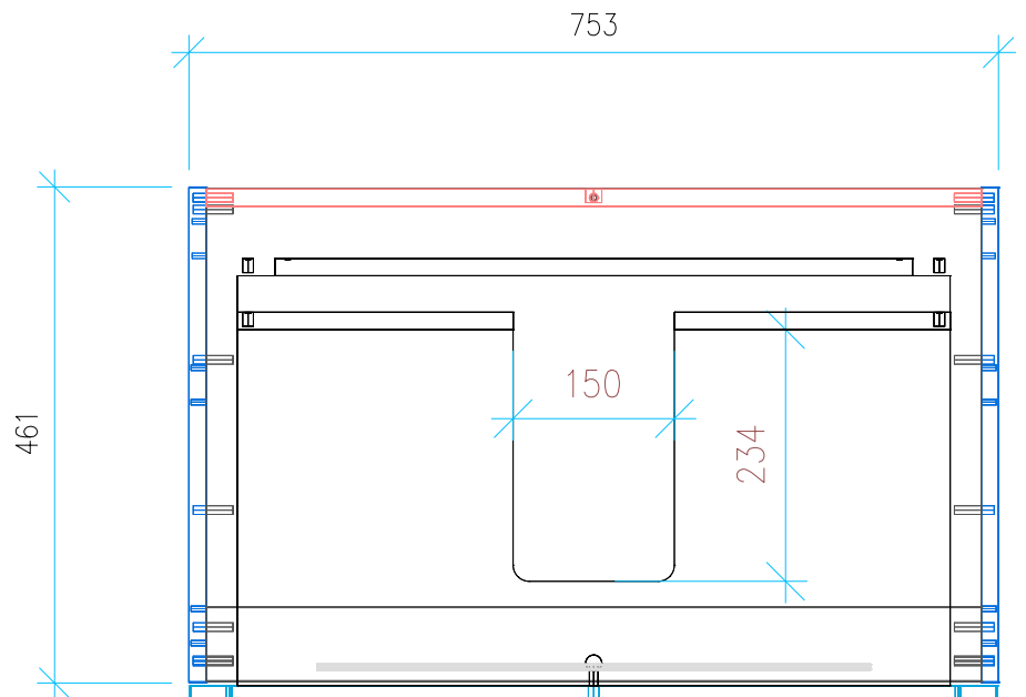
Ansicht 2 / Draufsicht
