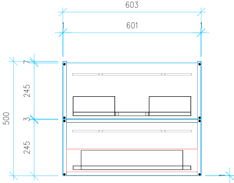
Ansicht 4 / Vorderansicht
