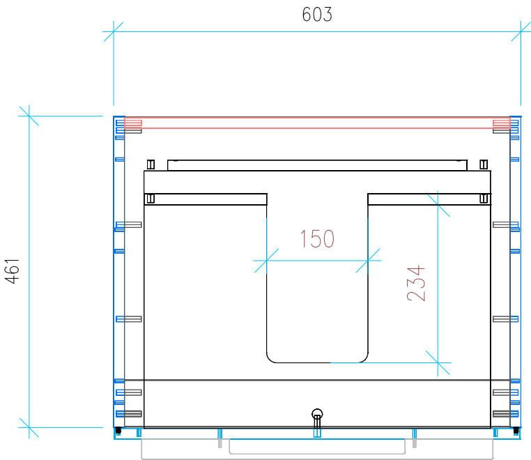
Ansicht 2 / Draufsicht
