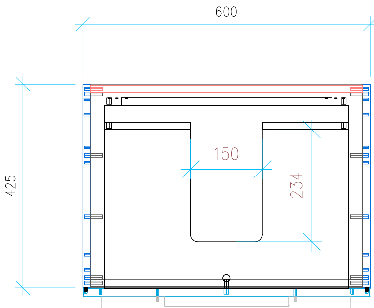
Ansicht 2 / Draufsicht
