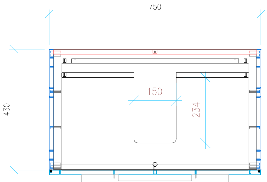
Ansicht 2 / Draufsicht
