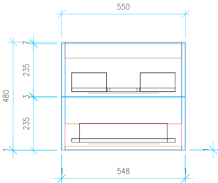
Ansicht 4 / Vorderansicht
