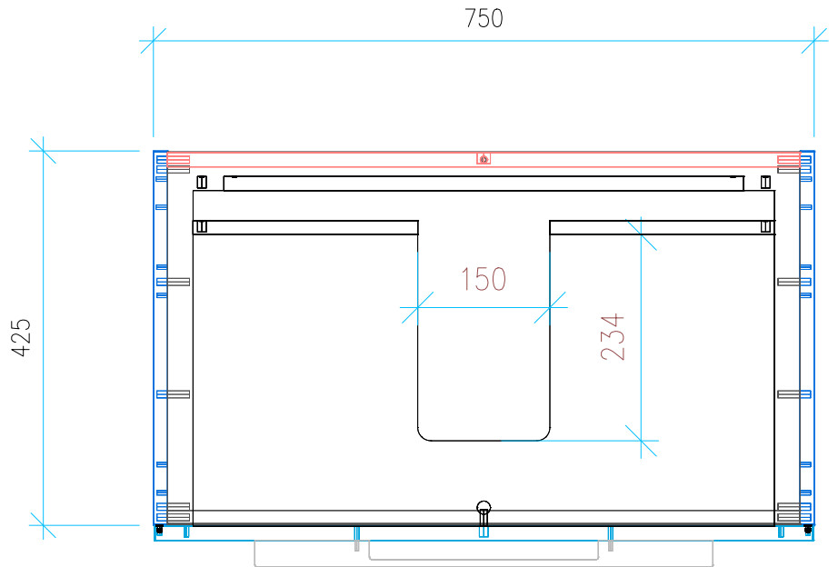
Ansicht 2 / Draufsicht
