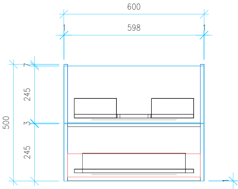
Ansicht 4 / Vorderansicht
