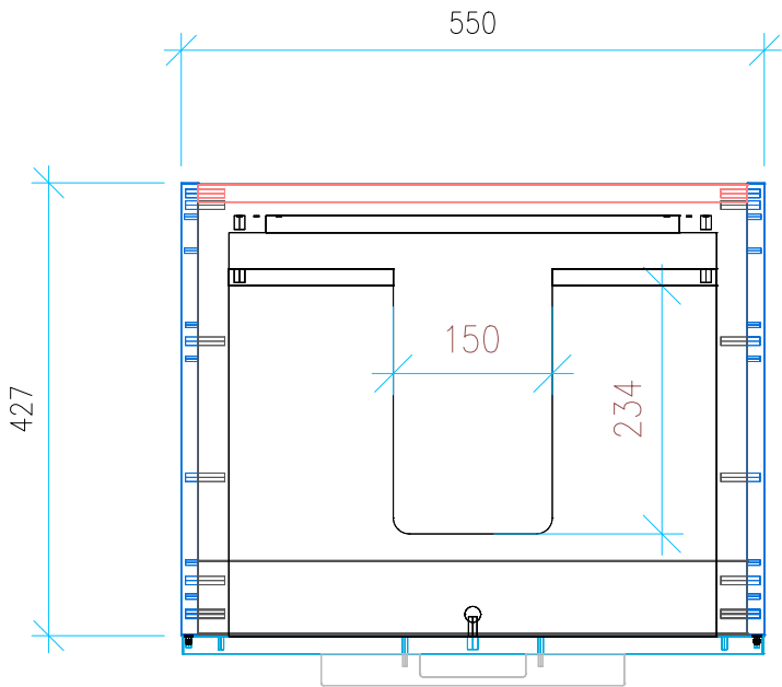
Ansicht 2 / Draufsicht
