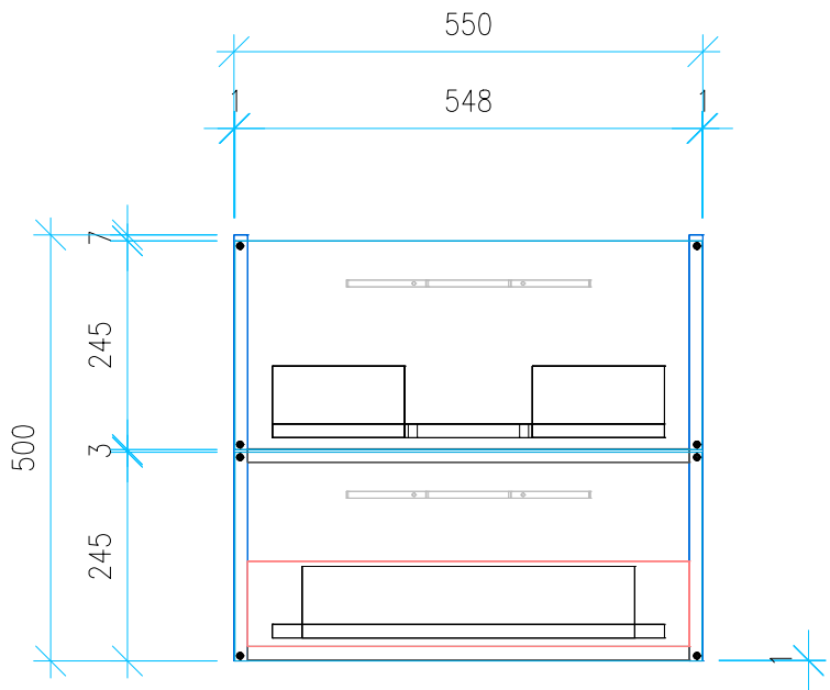
Ansicht 4 / Vorderansicht
