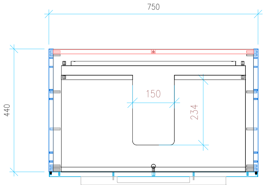
Ansicht 2 / Draufsicht
