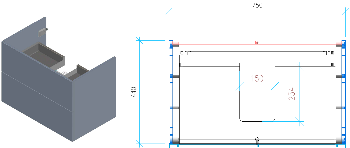
Ansicht 1 / 3D
