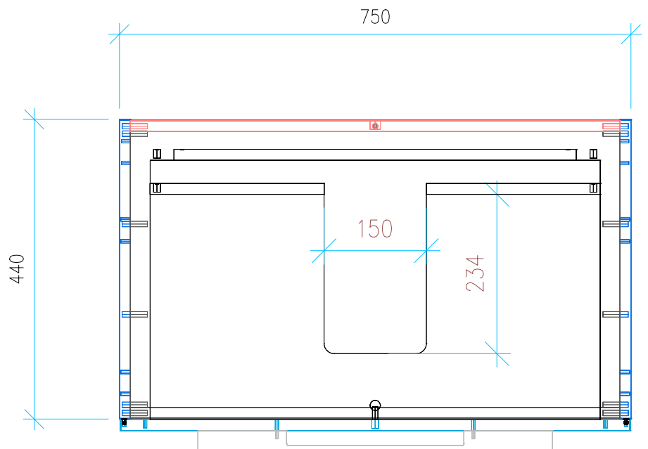
Ansicht 2 / Draufsicht
