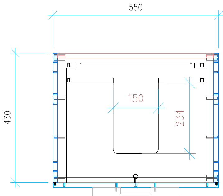
Ansicht 2 / Draufsicht
