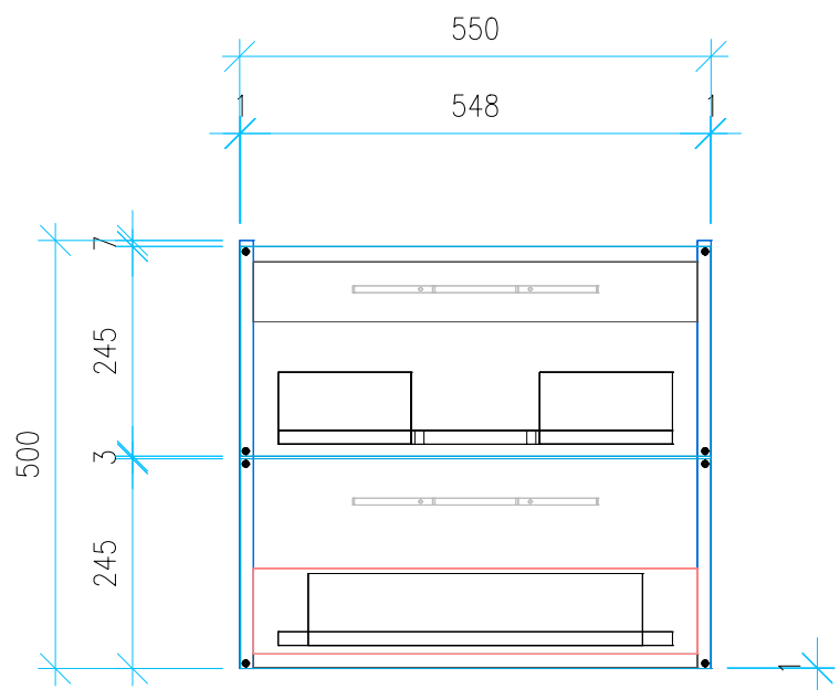
Ansicht 4 / Vorderansicht
