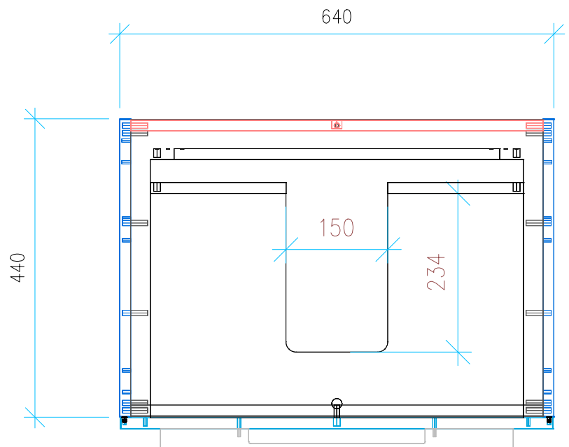
Ansicht 2 / Draufsicht
