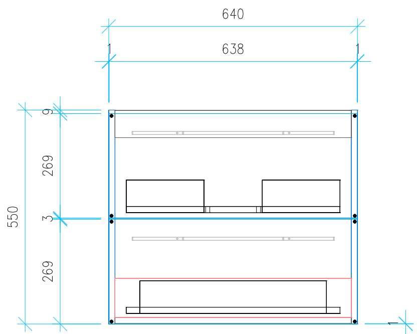
Ansicht 4 / Vorderansicht
