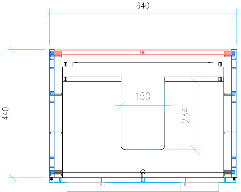
Ansicht 2 / Draufsicht
