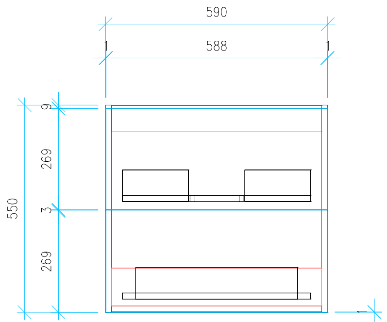
Ansicht 4 / Vorderansicht
