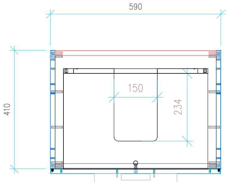
Ansicht 2 / Draufsicht
