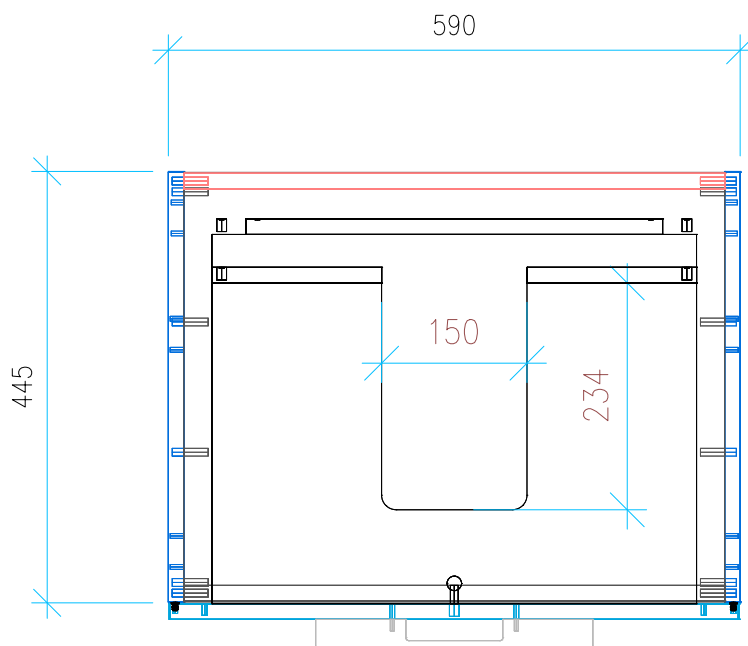
Ansicht 2 / Draufsicht
