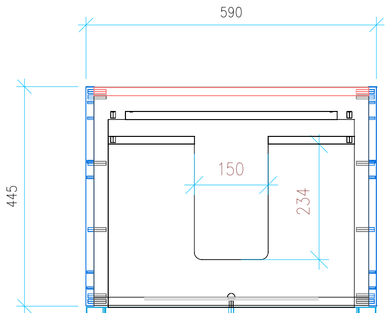
Ansicht 2 / Draufsicht
