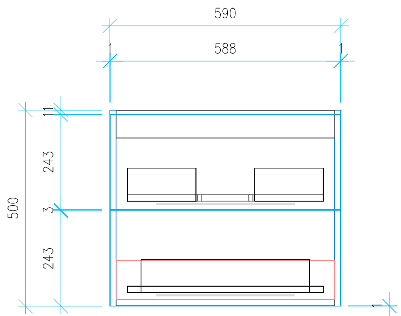
Ansicht 4 / Vorderansicht
