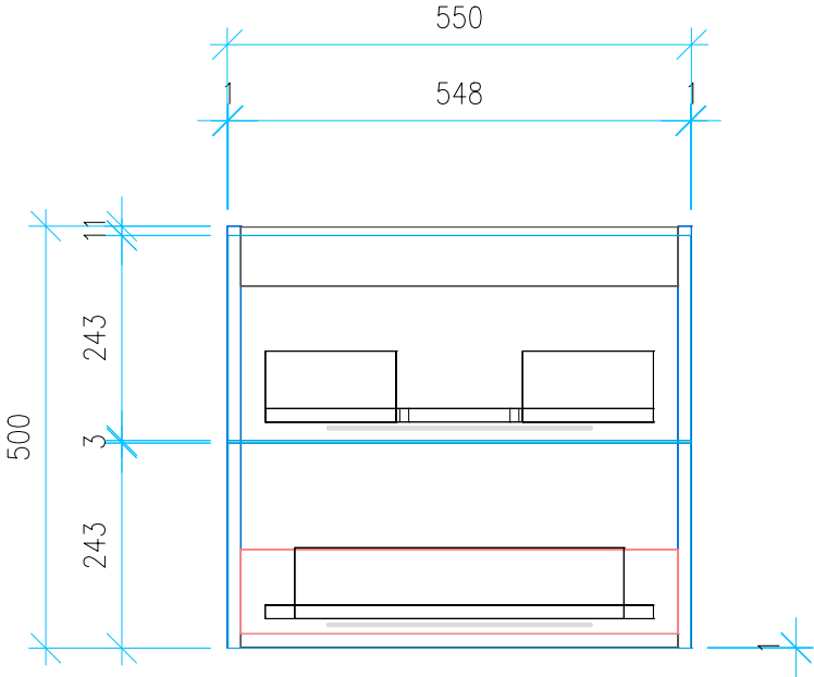
Ansicht 4 / Vorderansicht
