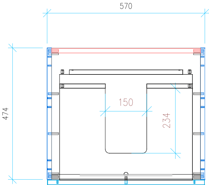
Ansicht 2 / Draufsicht
