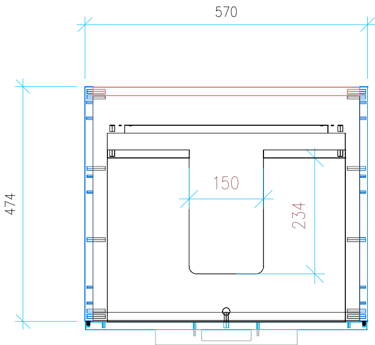
Ansicht 2 / Draufsicht
