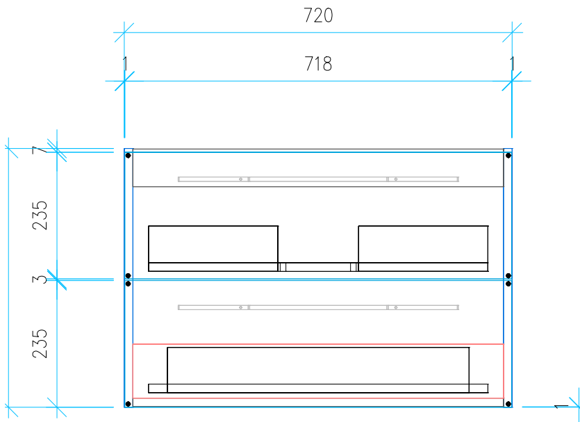
Ansicht 4 / Vorderansicht
