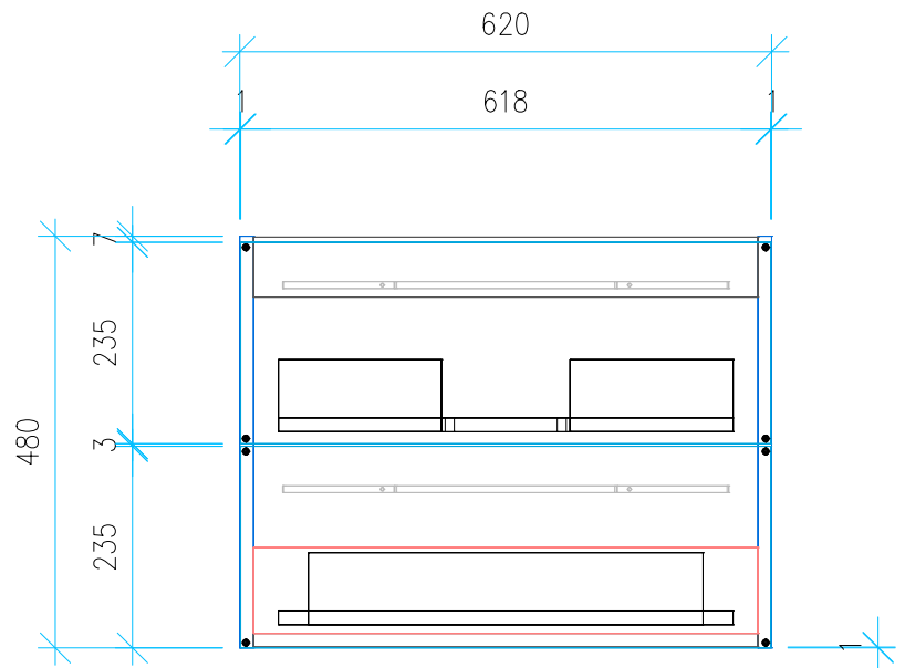
Ansicht 4 / Vorderansicht
