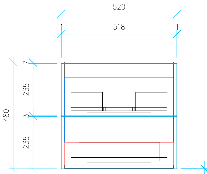
Ansicht 4 / Vorderansicht
