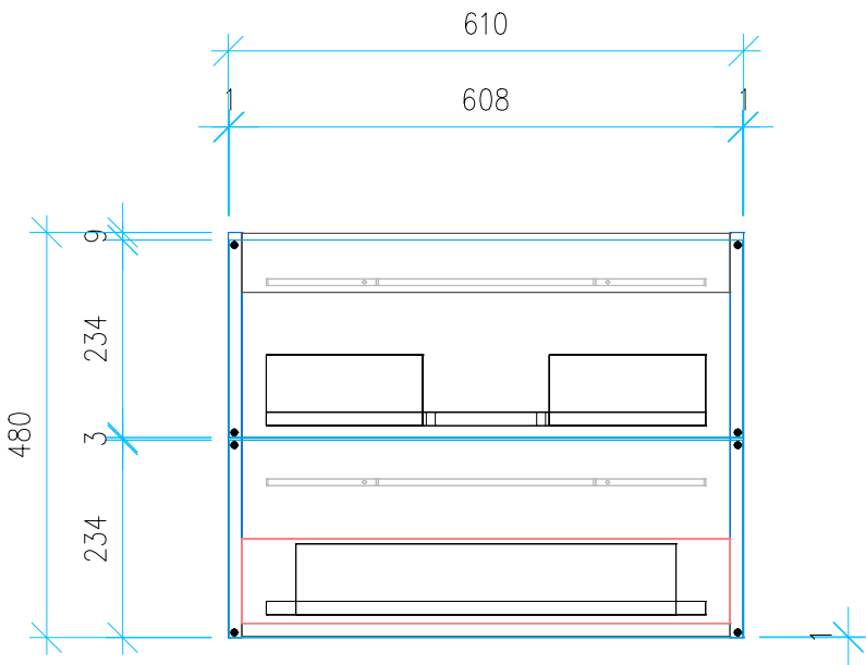
Ansicht 4 / Vorderansicht
