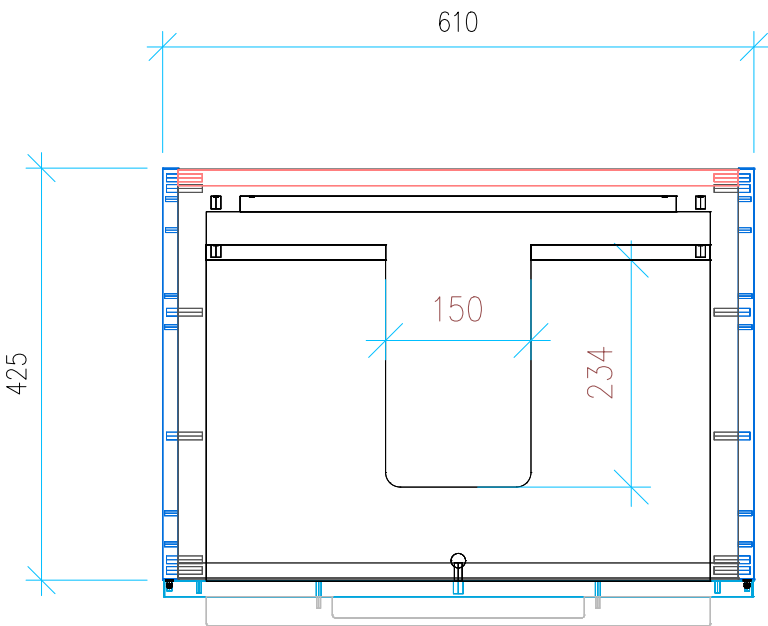
Ansicht 2 / Draufsicht
