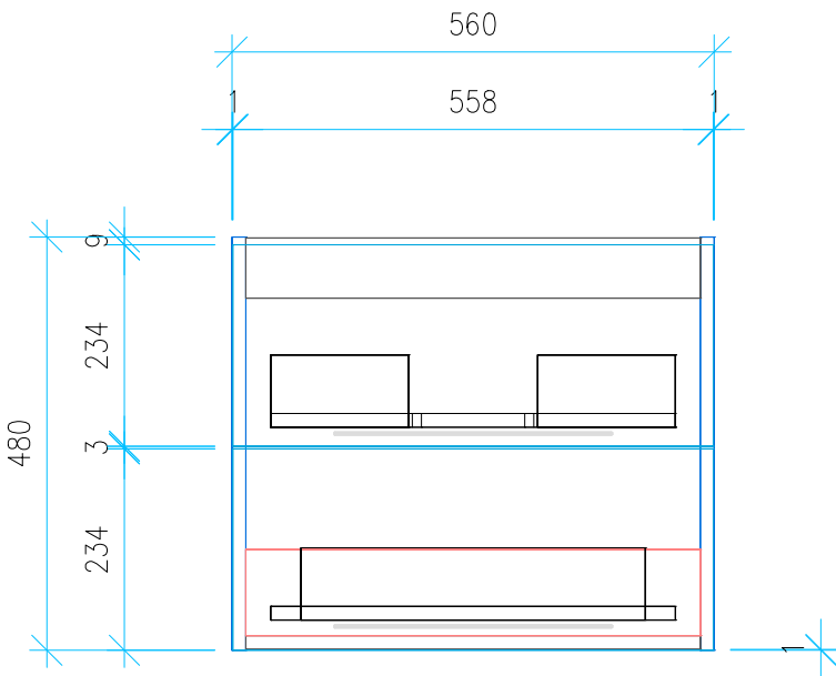
Ansicht 4 / Vorderansicht
