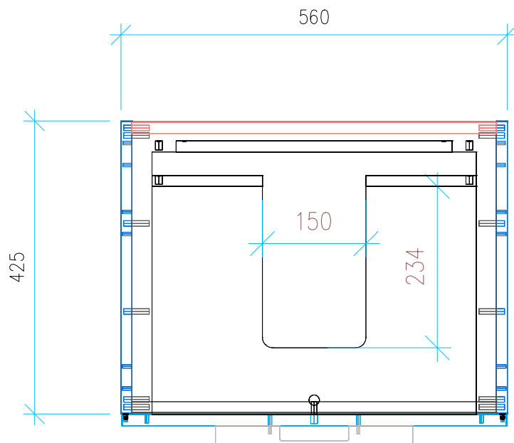
Ansicht 2 / Draufsicht
