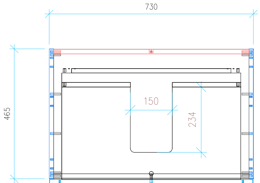
Ansicht 2 / Draufsicht
