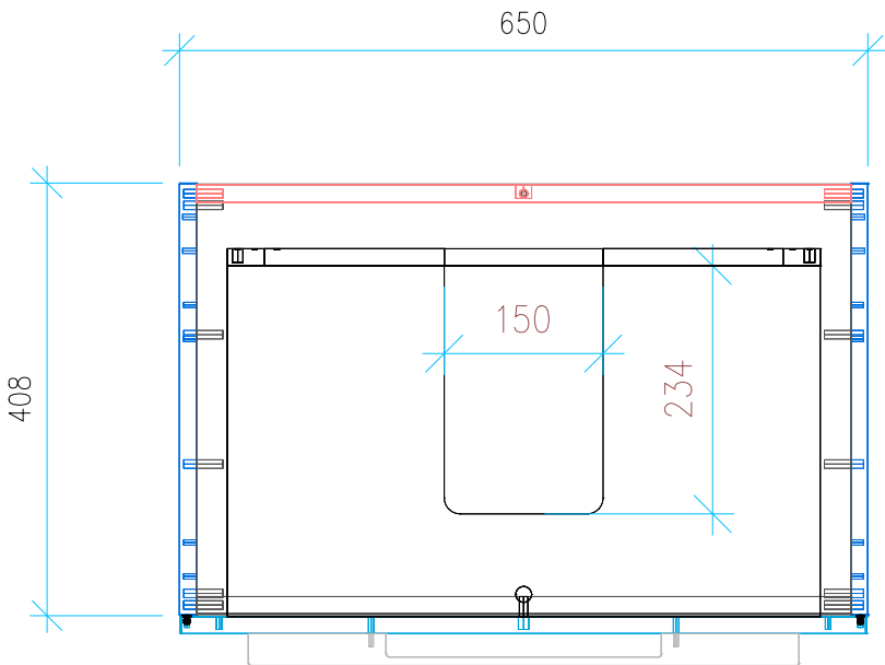
Ansicht 2 / Draufsicht
