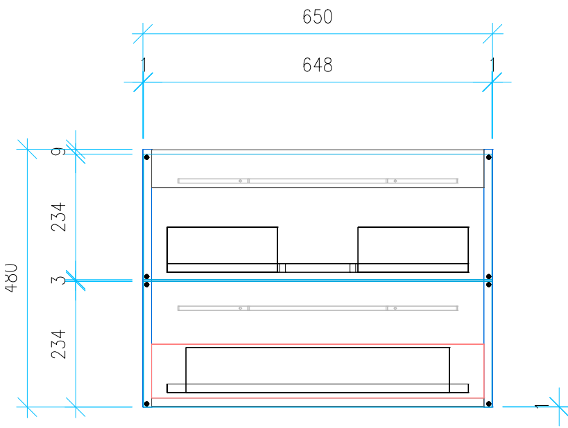
Ansicht 4 / Vorderansicht
