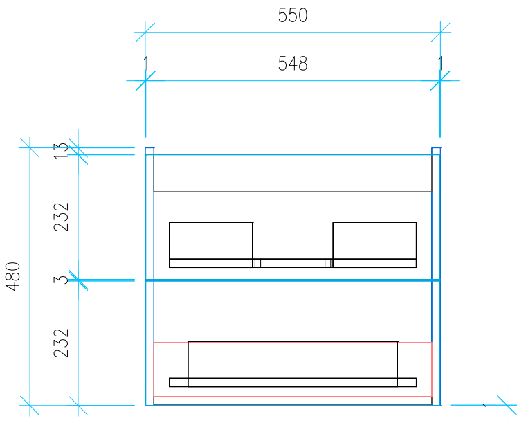
Ansicht 4 / Vorderansicht
