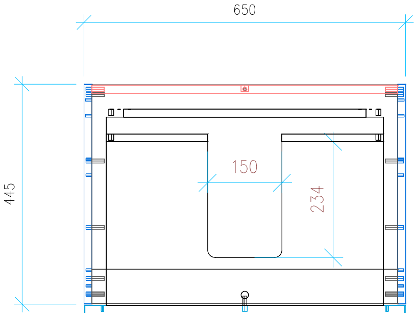
Ansicht 2 / Draufsicht
