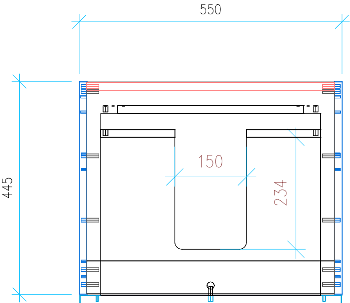
Ansicht 2 / Draufsicht
