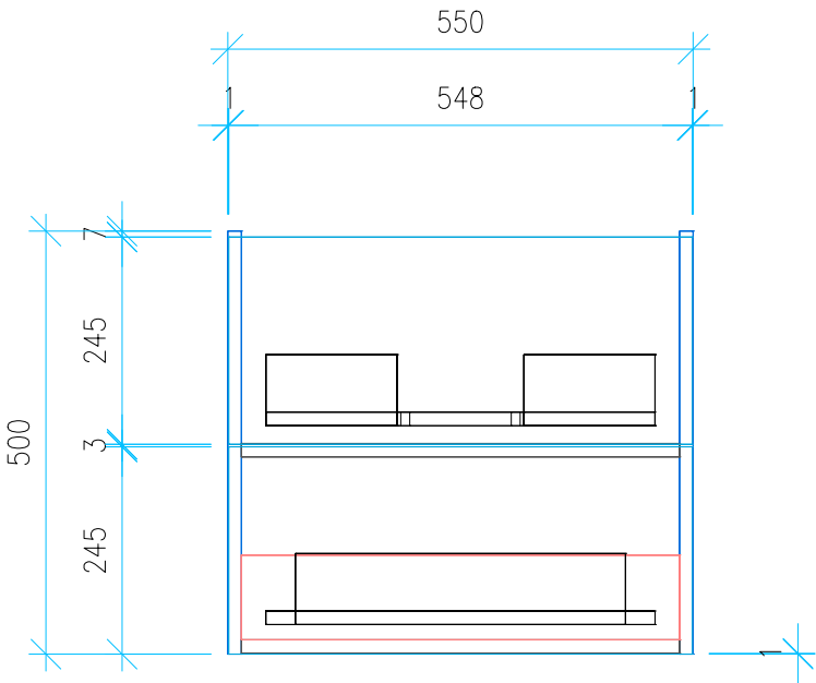
Ansicht 4 / Vorderansicht
