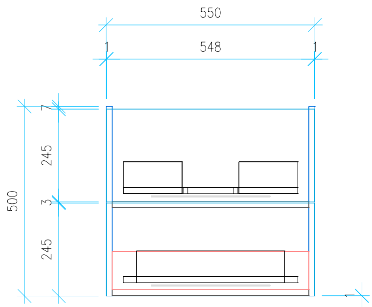
Ansicht 4 / Vorderansicht
