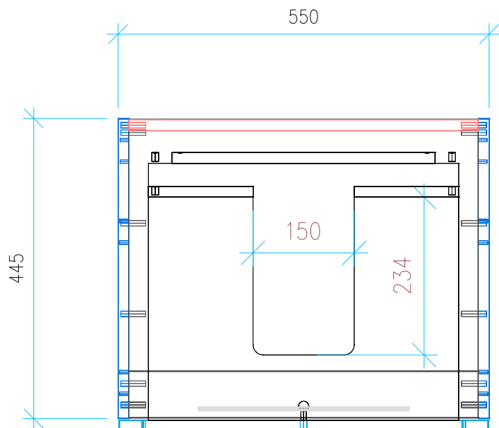
Ansicht 2 / Draufsicht
