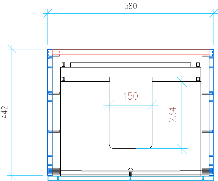
Ansicht 2 / Draufsicht
