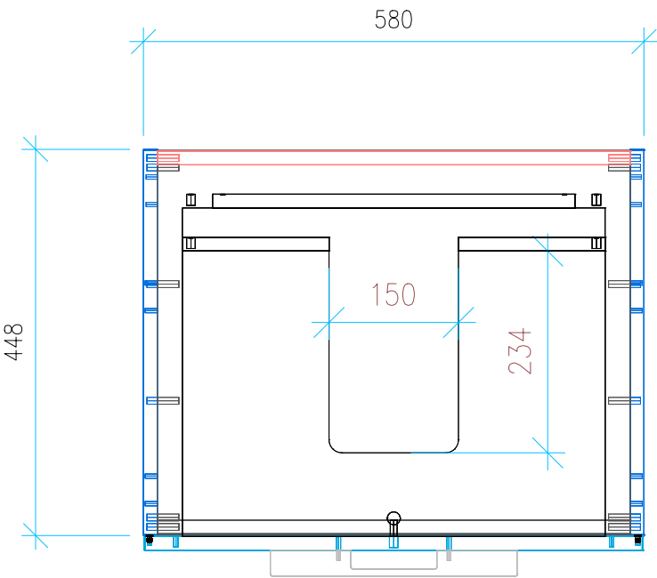
Ansicht 2 / Draufsicht
