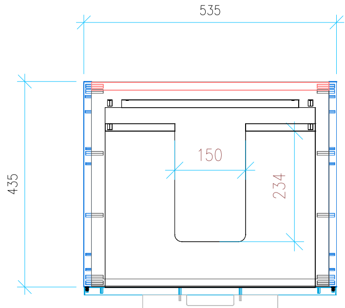
Ansicht 2 / Draufsicht
