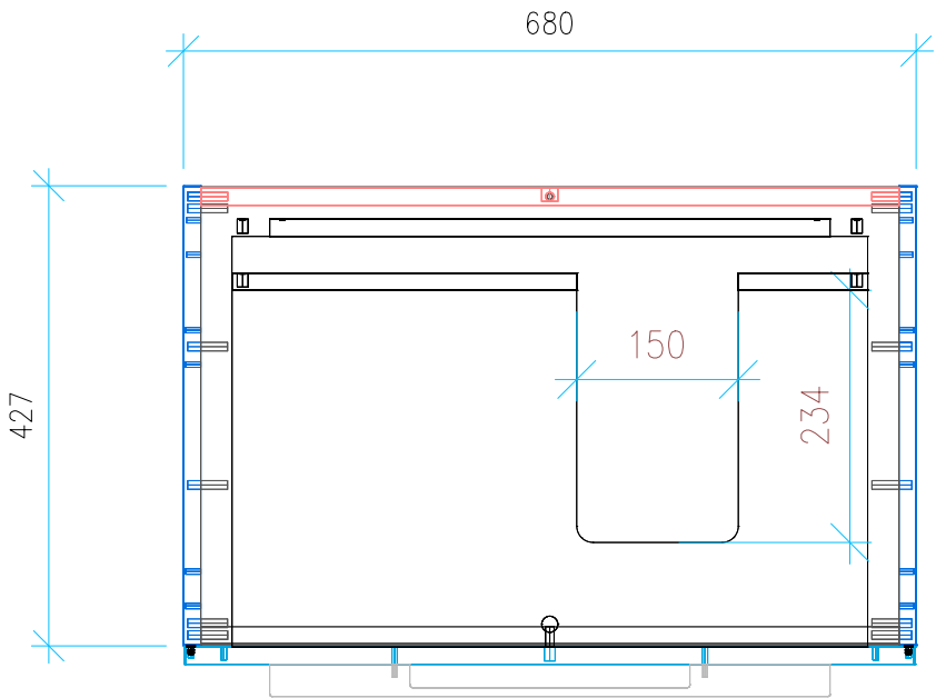
Ansicht 2 / Draufsicht
