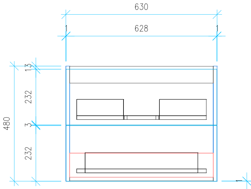
Ansicht 4 / Vorderansicht
