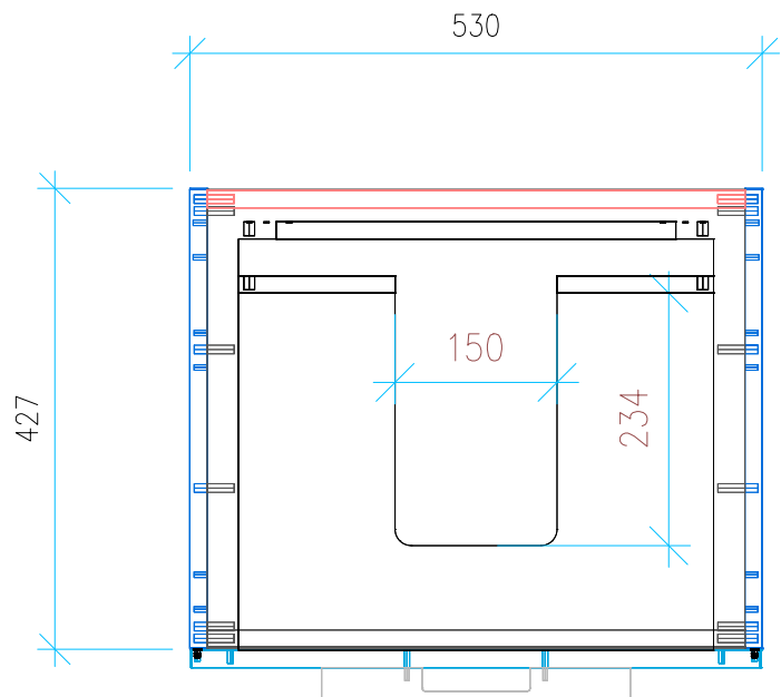
Ansicht 2 / Draufsicht
