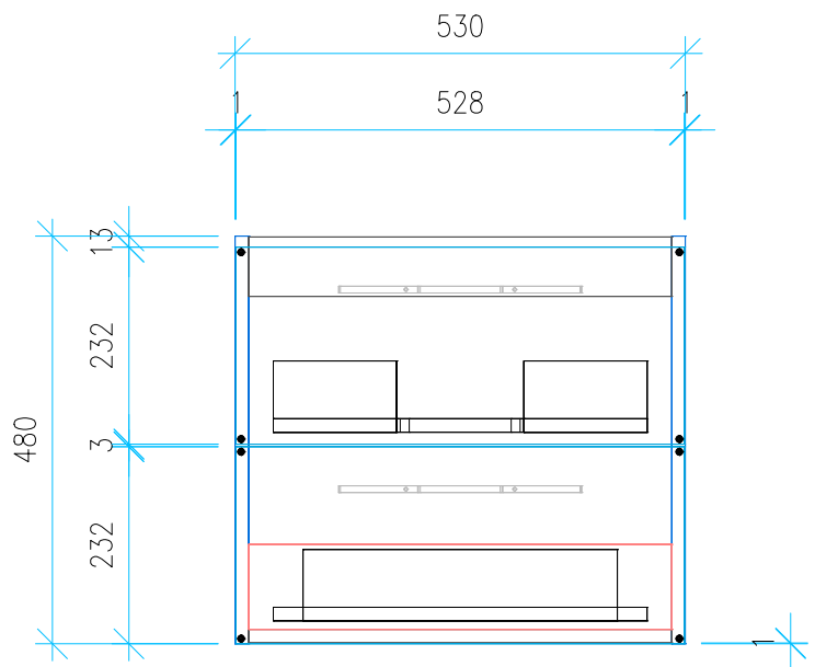
Ansicht 4 / Vorderansicht
