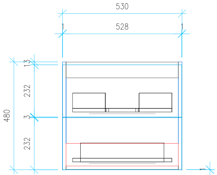
Ansicht 4 / Vorderansicht
