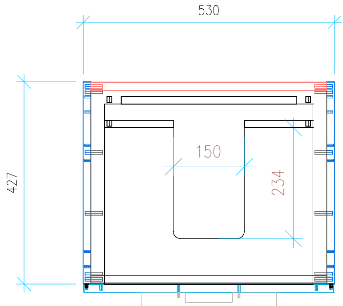
Ansicht 2 / Draufsicht
