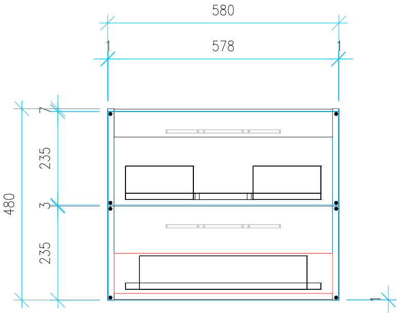
Ansicht 4 / Vorderansicht
