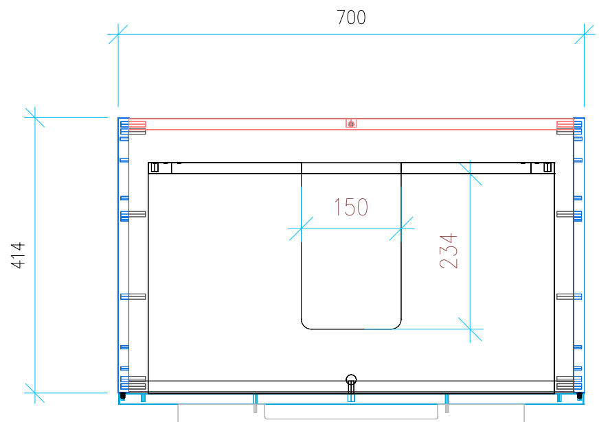
Ansicht 2 / Draufsicht
