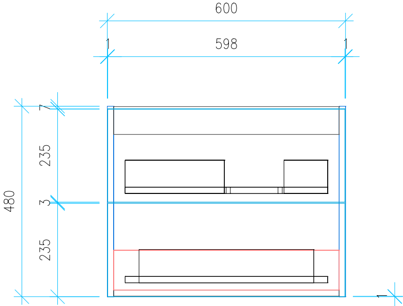
Ansicht 4 / Vorderansicht
