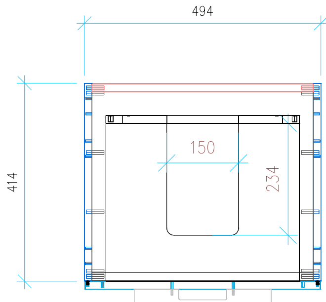
Ansicht 2 / Draufsicht
