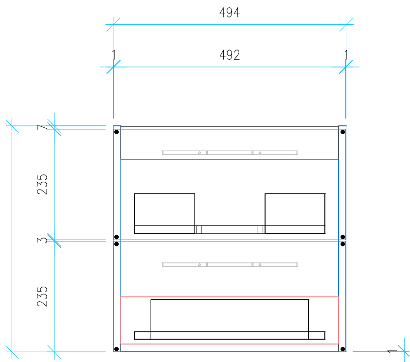
Ansicht 4 / Vorderansicht
