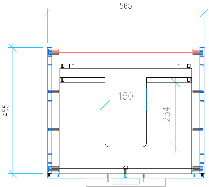
Ansicht 2 / Draufsicht
