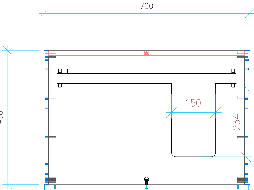
Ansicht 2 / Draufsicht
