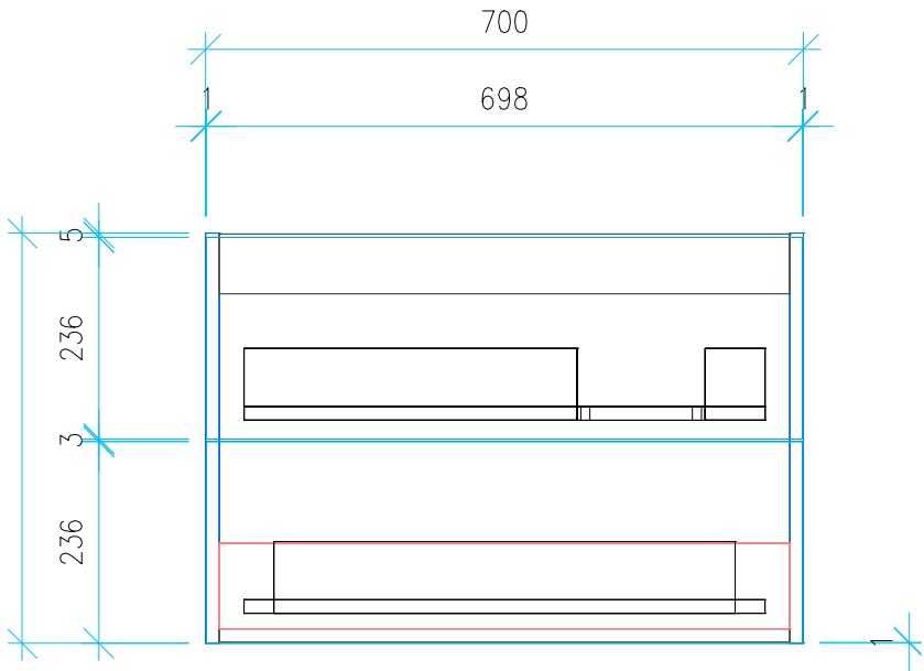
Ansicht 4 / Vorderansicht
