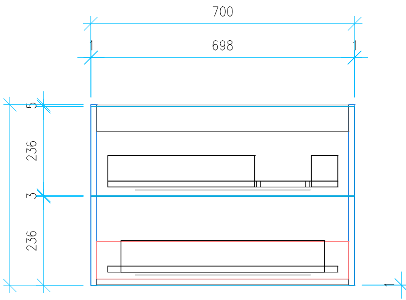
Ansicht 4 / Vorderansicht
