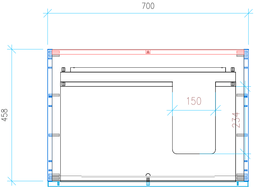
Ansicht 2 / Draufsicht
