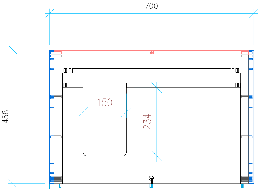
Ansicht 2 / Draufsicht
