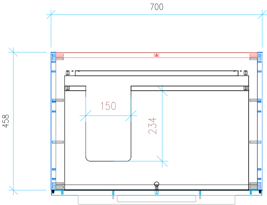
Ansicht 2 / Draufsicht
